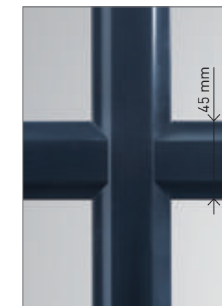
Inglesina ALLUMINIO - Disponibile in bianco, bicolore o monocolore Sezione 45x8 mm
