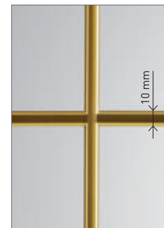
Inglesina OTTONE TRADI Sezione 10x8 mm
