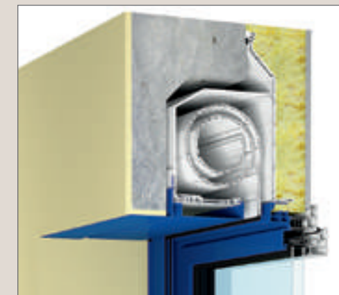
Il monoblocco ½ architrave
